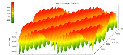
高速永磁电机2D时域扭矩分布
