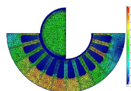
高速永磁电机电磁有限元分析
